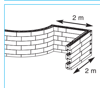
Les escaliers Piano 1,50 m et 2 m sont livrés avec des blocs cintrés.
