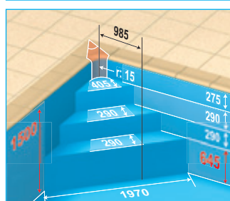
Escaliers d'angle
